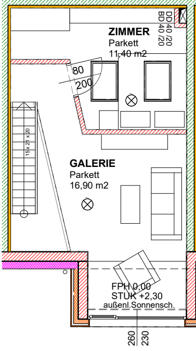
OBERGESCHOSS, M 1:100
