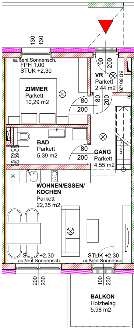
OBERGESCHOSS, M 1:100
