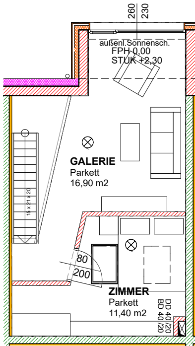
OBERGESCHOSS, M 1:100
