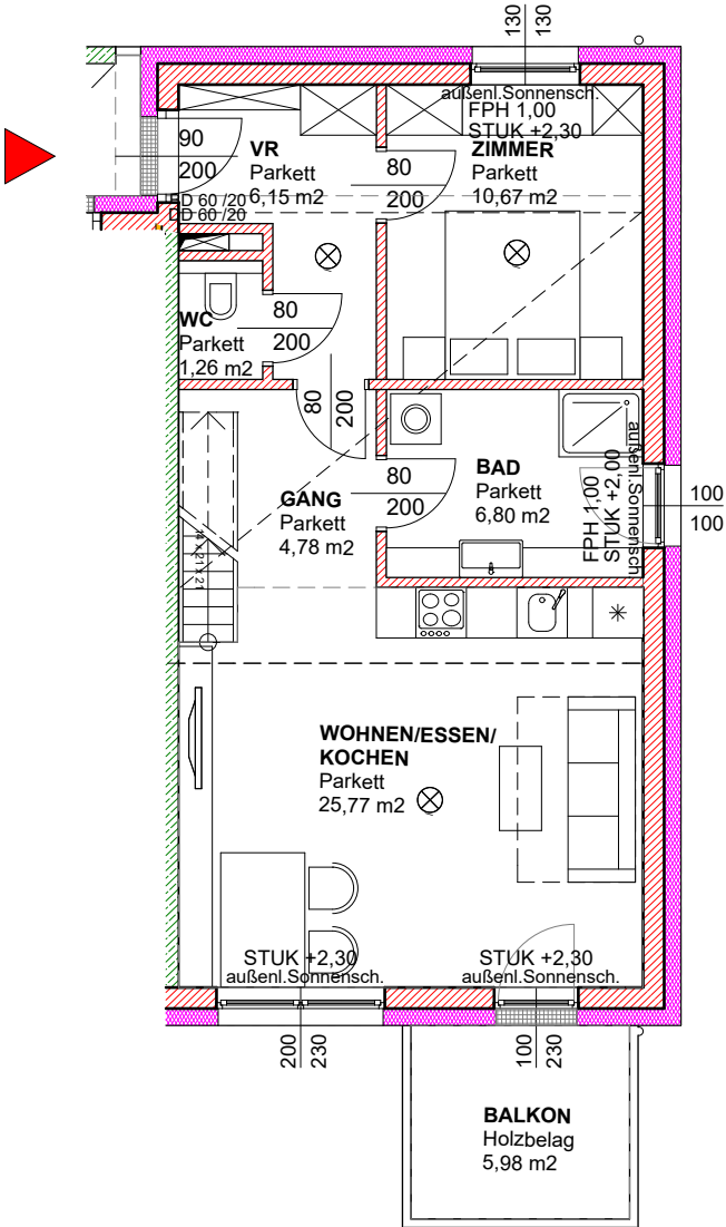
ERDGESCHOSS, M 1:100
