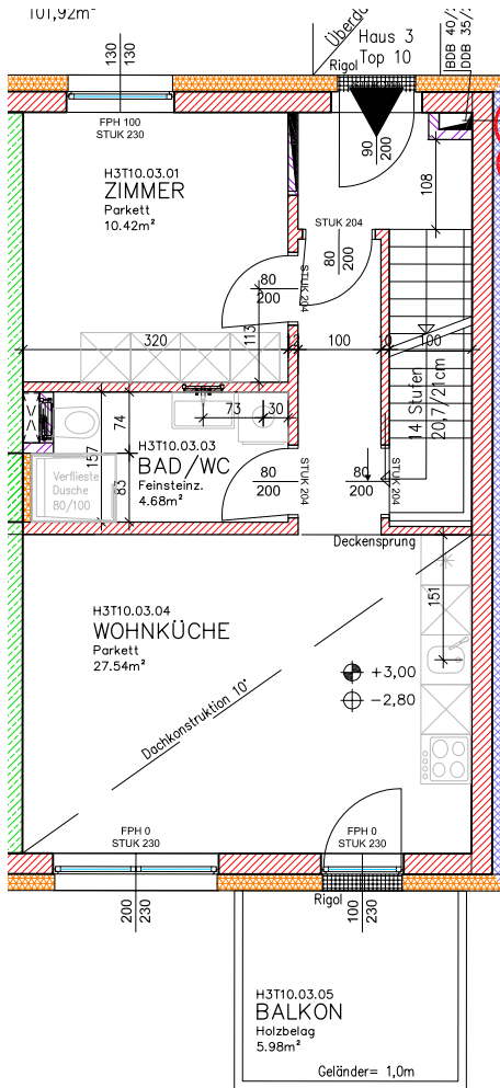
1. OBERGESCHOSS
