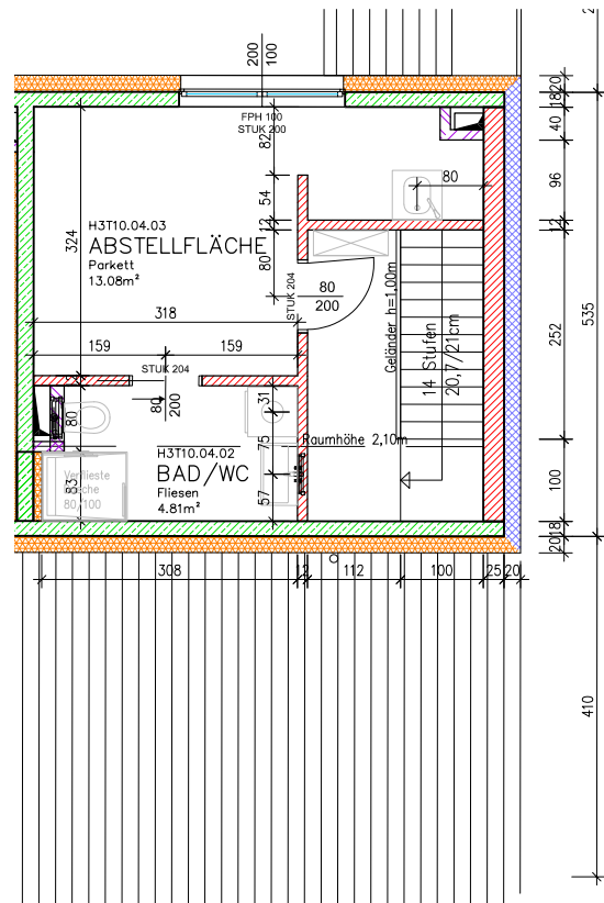
DACHBODEN
