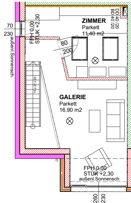
OBERGESCHOSS, M 1:100
