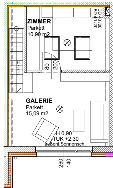
OBERGESCHOSS, M 1:100
